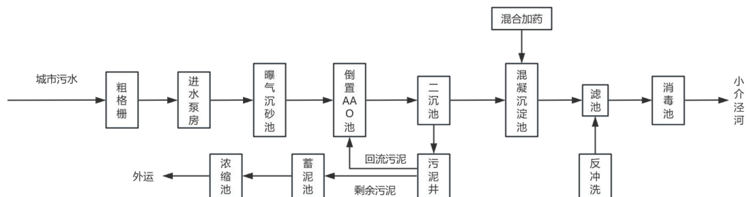
图 4-2 昆山市锦溪污水处理厂有限公司处理工艺
