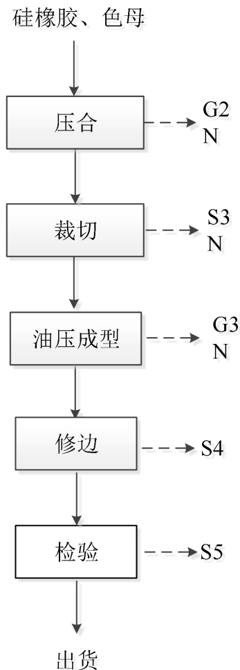
图 2-5 硅胶零部件工艺流程图
