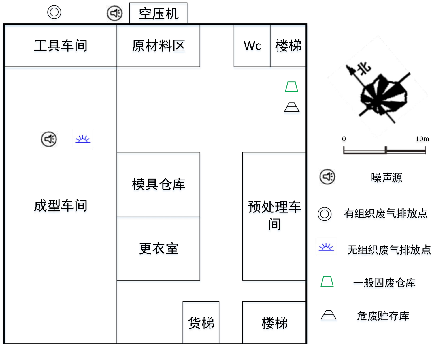
附图 5-2 建设项目 1 楼车间平面布置图
