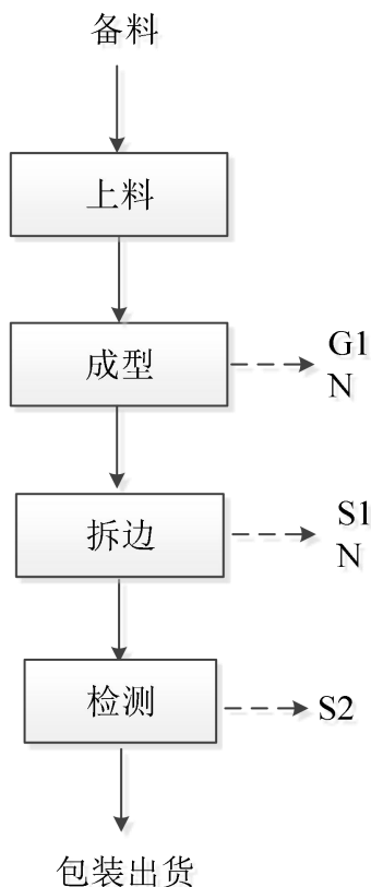
图 2-4 硅胶制品工艺流程图
