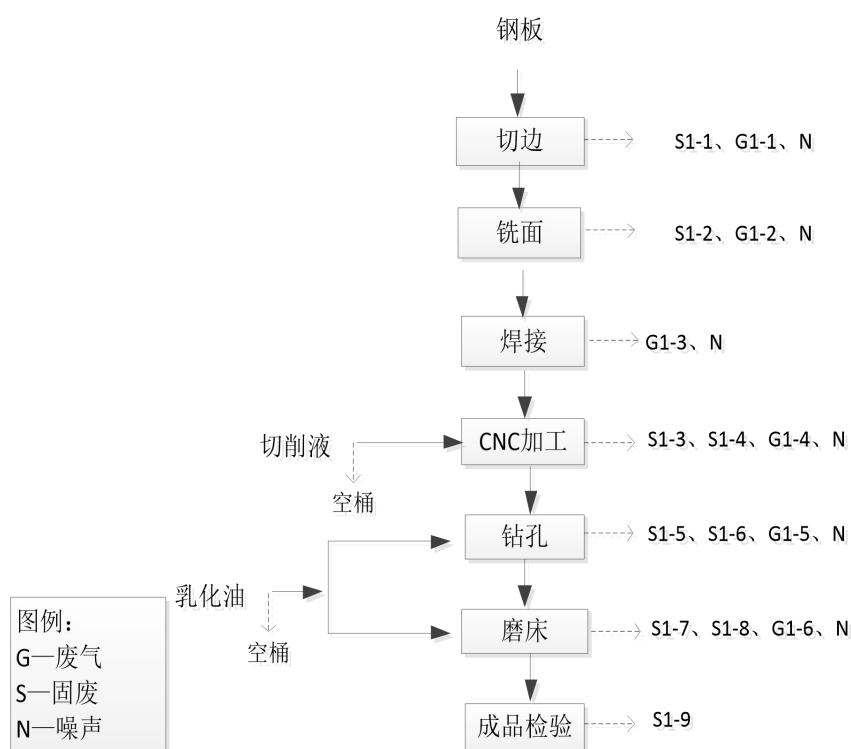
图 5-1 模具墙板生产工艺流程图
