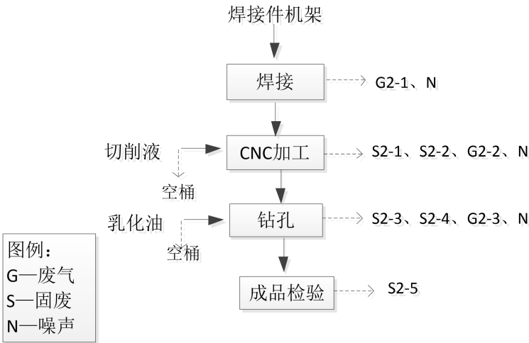
图 5-2 焊接件生产工艺流程图
