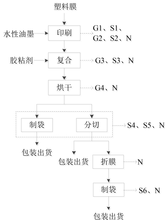
图 3.5-1 塑料袋生产工艺流程图
