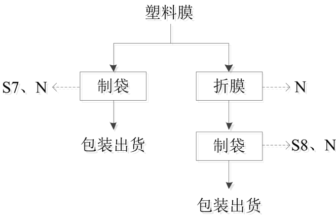
图 3.5-2 塑料膜生产工艺流程图
