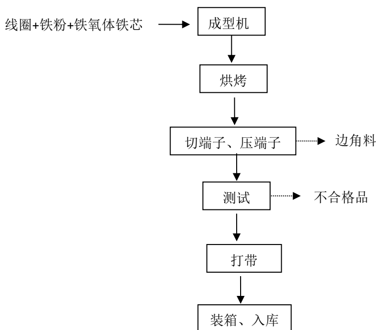
图 3.5-1 电感器生产工艺流程及产污环节图
