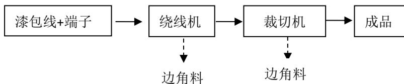
图 3.5-4 线圈生产工艺流程及产污环节图
